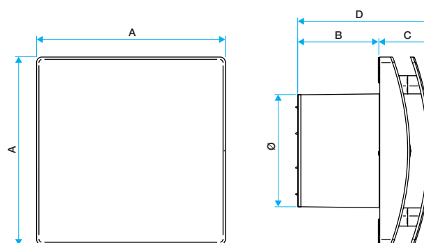
GRAPHIC Encombrement
