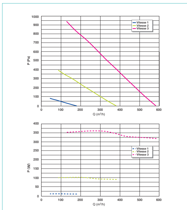
Constant snelheid
