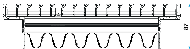
Gridlined floor avec registre monté
