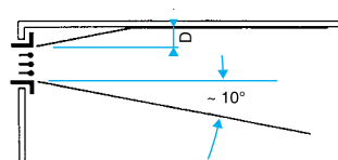
A) Soufflage avec effet de plafond où D inférieur ou égal à 30 cm.
