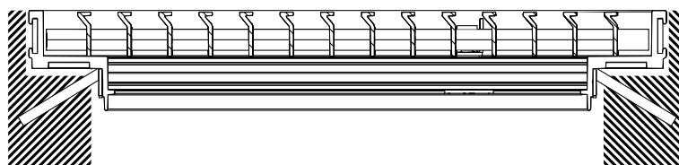
Gridlined floor avec ses pattes de scellement
