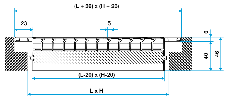
Gridlined wall double déflexion
