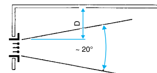
B) Soufflage sans effet de plafond où D supérieur à 30 cm.
