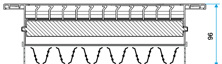
Gridlined wall double déflexion avec registre monté
