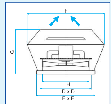
THELIA Verticale luchtstroom
